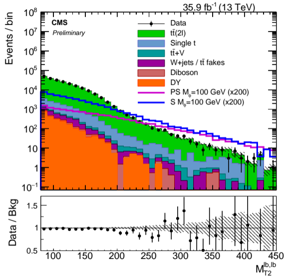
(b) M_{T2}^{\text{lb,lb}}
