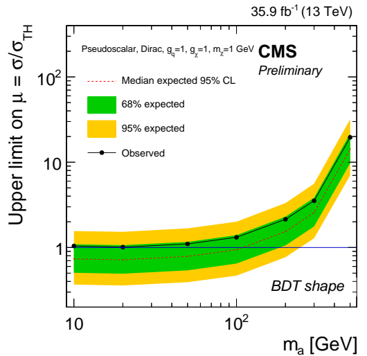
(d) BDT discriminant: pseudoscalar mediator
