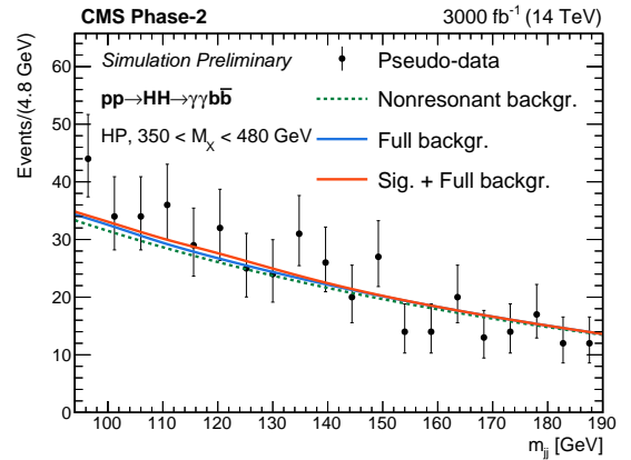
(d) m_{jj} , medium mass category
