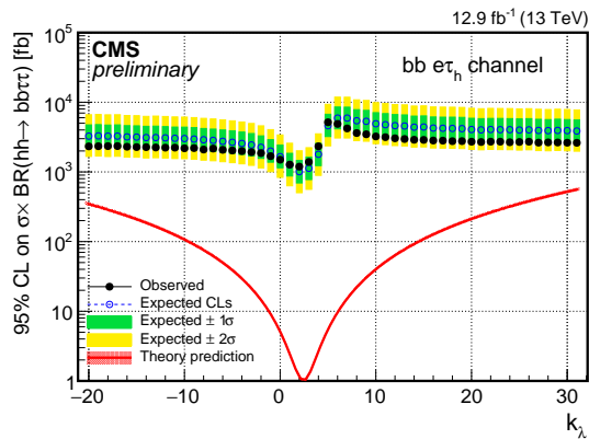
(b) bbe\tau_h
