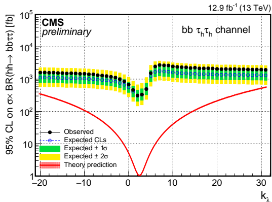
(c) bb\tau_h\tau_h
