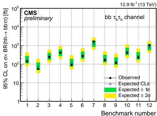
(c) bb\tau_h\tau_h
