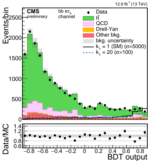
(b) bbe\tau_h
