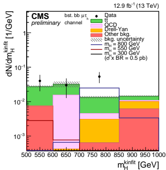
(g) \mu\tau_h : boosted
