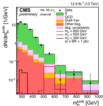
(d) \mu\tau_h : resolved 2b
