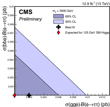
(d) m_\phi = 2900 GeV
