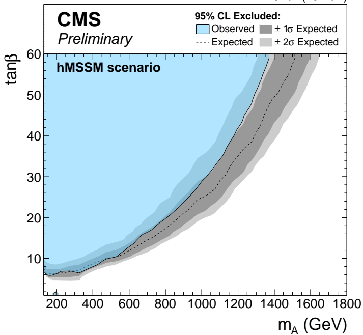
(b) hMSSM
