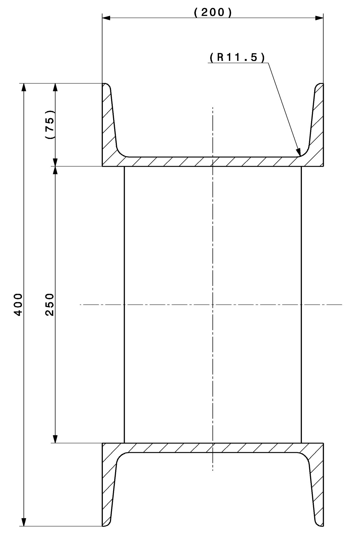
Section view A-A Scale: 1:2
