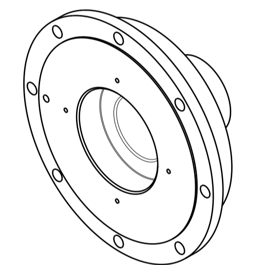
Vue isométrique Echelle : 1:1
