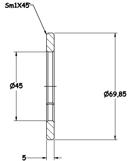
A-A (1:1)
