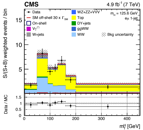
(d) GF 1-jet off-shell
