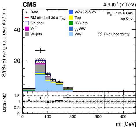
(a) GF 0-jet on-shell
