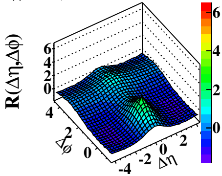
(a) PYTHIA \sqrt{s} = 0.9\text{TeV}
