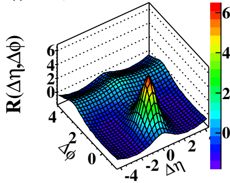
(c) PYTHIA \sqrt{s} = 7\text{TeV}
