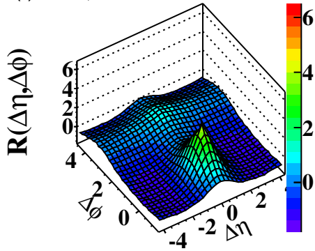
(b) PYTHIA \sqrt{s} = 2.36\text{TeV}
