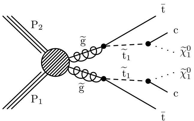
(d) T5ttcc
