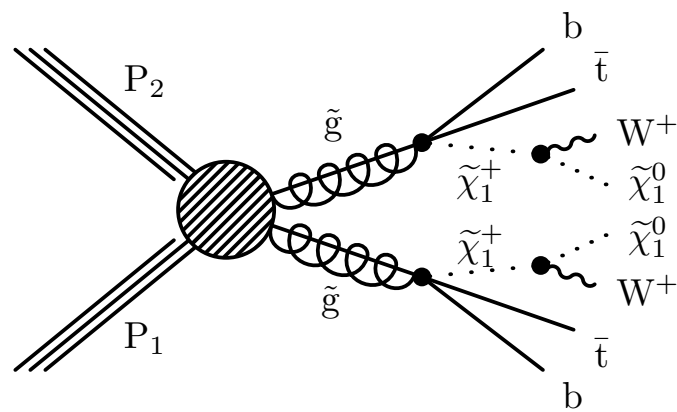
(b) T5ttbbWW
