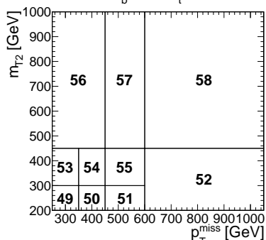
N_b=1 & N_t \geq 3
