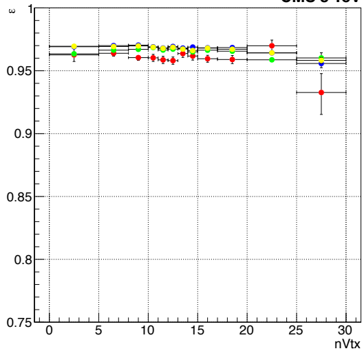
CMS 8 TeV
