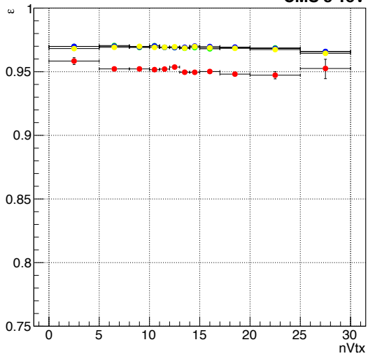
CMS 8 TeV
